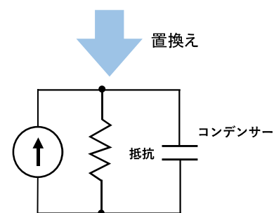
図2: 熱等価回路
